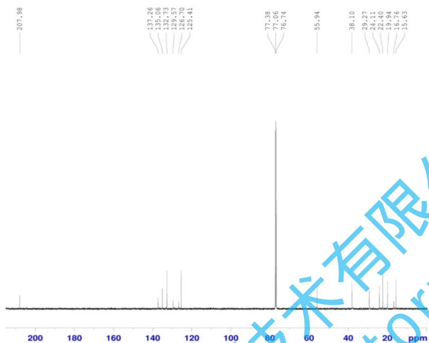
附 ^{13}\text{C} -NMR 图
