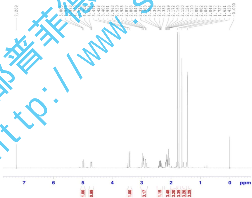
附 ^1\text{H} -NMR 图
